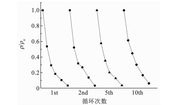
图 10 不同循环次数下橙黄 II 的降解曲线 Fig. 10 Orange II degradation curves under different cycles
