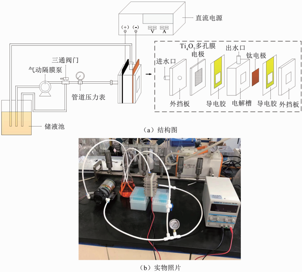
图 1 穿流-电催化氧化系统的结构与实物照片
